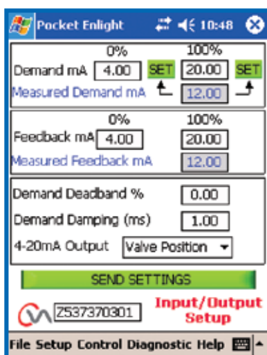
Настройка 4-20 мА
