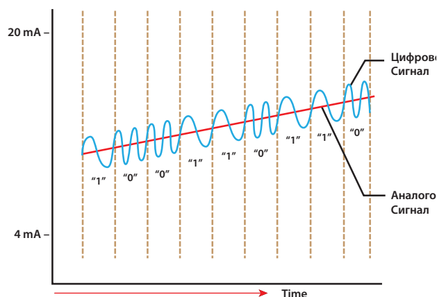
Рис. 4: Принцип FSK (источник: HART ® )
