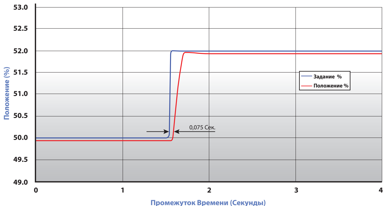
Rotork CVA Реакция на скачек T86b = 0.175 сек.
